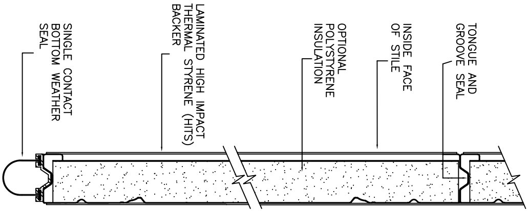
— SECTION THRU DOOR —
